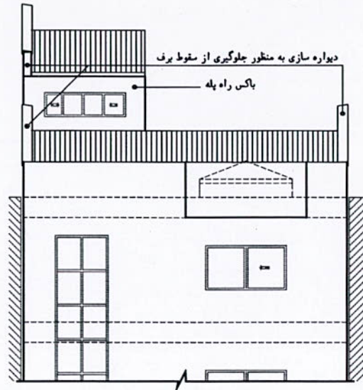
نمای اصلی
