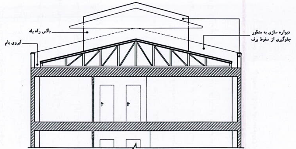
مقطع C-C
