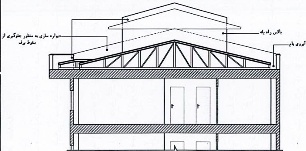
مقطع B-B
